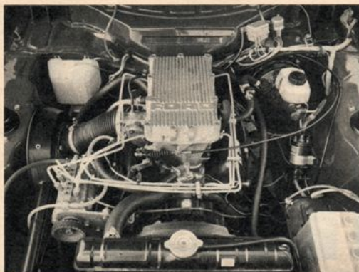
Der Einspritzmotor des Capri RS zeichnet sich durch eindrucksvolle Elastizität und hohe Leistung aus. Die klar gezeichneten Rundinstrumente werden vom Lenkrad teilweise verdeckt.
